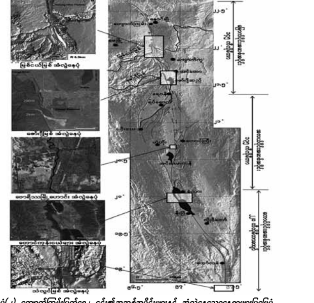
ပုံ(၂) ကျောက်ကြမ်းပြတ်ရွေ့၊ ၎င်း၏ အဆစ်အပိုင်းများနှင့် အလွဲနေသောနေရာများပြမြေပုံ
