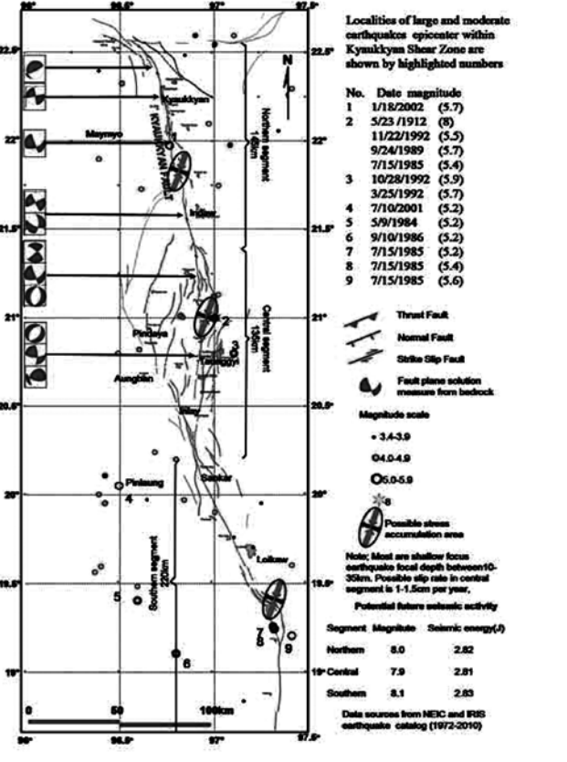
ပုံ(၃) ကျောက်ကြမ်းပြတ်ရွေ့နှင့် ၎င်း၏ အဆစ်အပိုင်းများ၊ မြေငလျင်ဗဟိုချက်များ၊ အမြင့်ဆုံးမြင့်နိုင်ခြေမြေငလျင်ပြင်းအားနှင့် မြေငလျင်ဗဟိုချက်ဖြစ်နိုင်ခြေရှိသော နေရာများပြမြေပုံ
