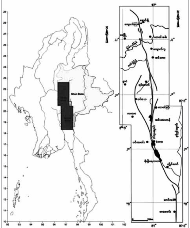
ပုံ(၁) ကျောက်ကြမ်းပြတ်ရွေ့၏ တည်နေရာပြမြေပုံ
