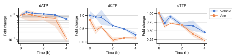
(f) dNTPs
