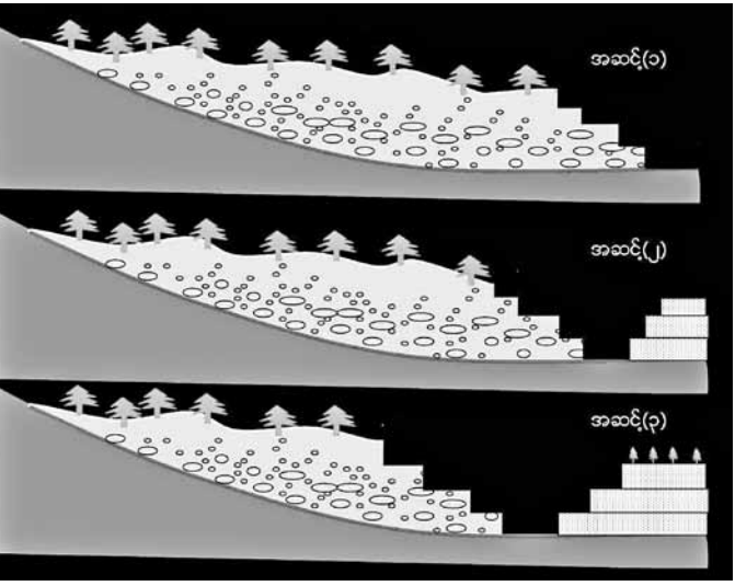
အကြံပြုတူးဖော်ရေးစနစ် အဆင့်ဆင့်ပြပုံ
