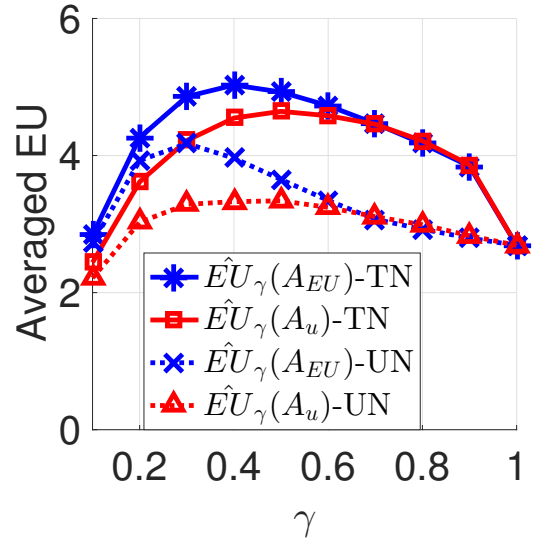
(d) n = 30, \kappa = 4, \Delta c = 0.5
